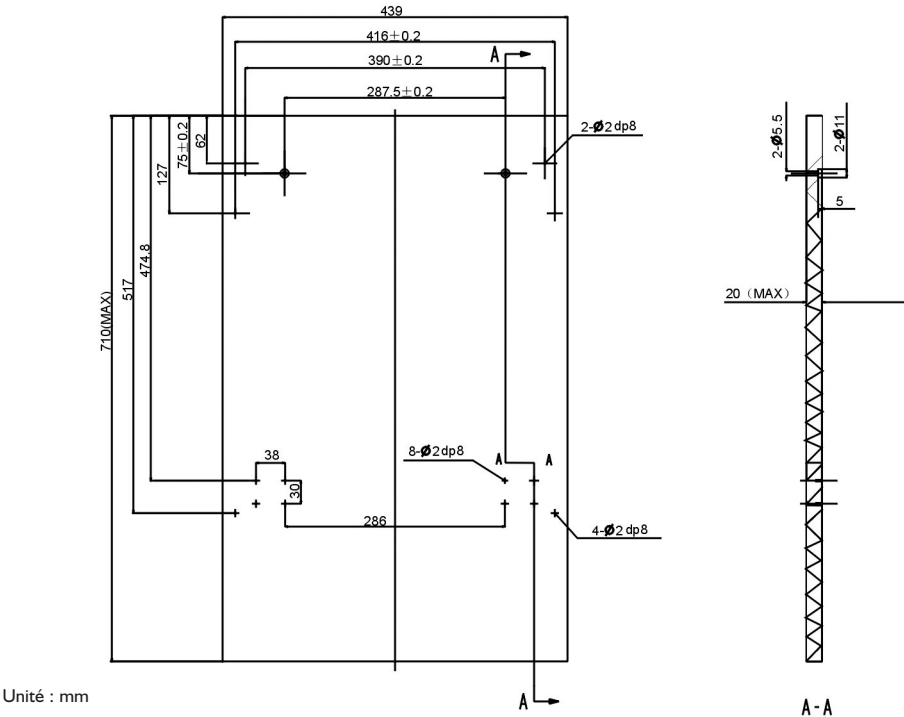
Figure 3 Le panneau décoratif doit être réalisé en respectant les dimensions illustrées.
