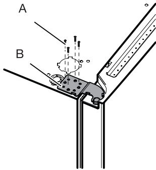
A. 5 mm socket wrench B. Top Hinge
