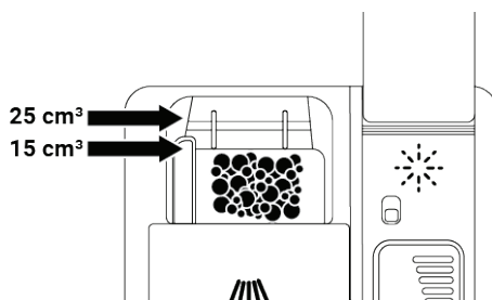
Darstellung 5.5.2: Das Befüllen des Spülmittels
