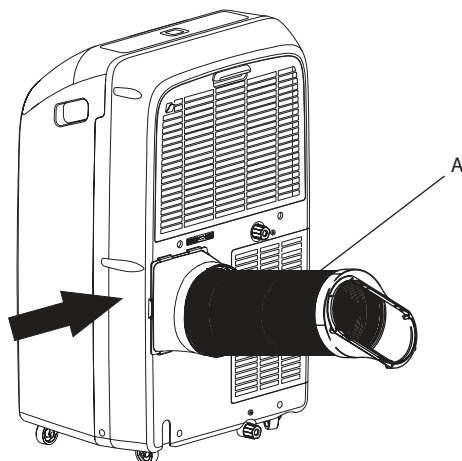
A. Zostava pružnej odvádzacej hadice
