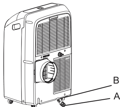
A. Hlavný kryt výpustu B. Hlavná vypúšťacia zátku
