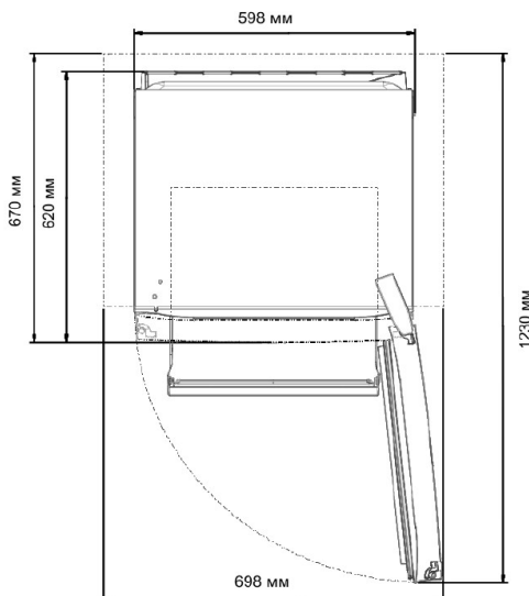
Муздаткыч прибордун жумушчу габариттери
