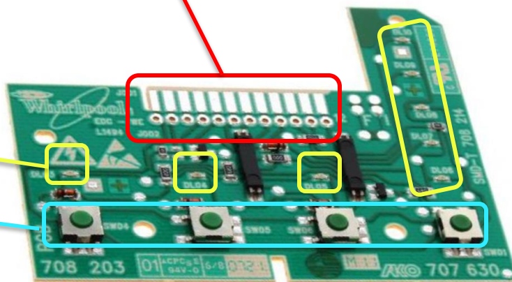
E3 - vue avant de la carte
