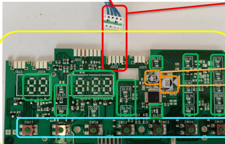
E8 - vue avant de la carte
