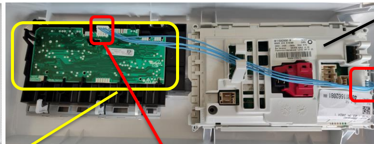
E8 - vue avant de la carte
